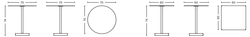
Ø70 x H74 cm
