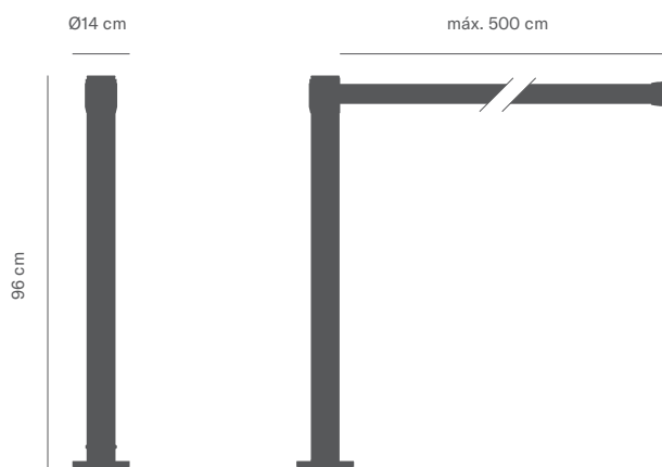
MAG Post
