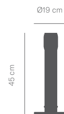
FIX MINI Post
