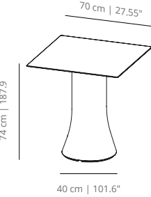
CAC70 table 7070 | 27 9 / 16 x 27 9 / 16
